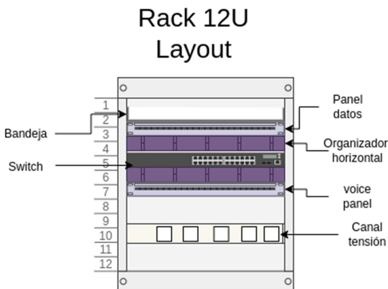
Ilustración 1: Layout interno
