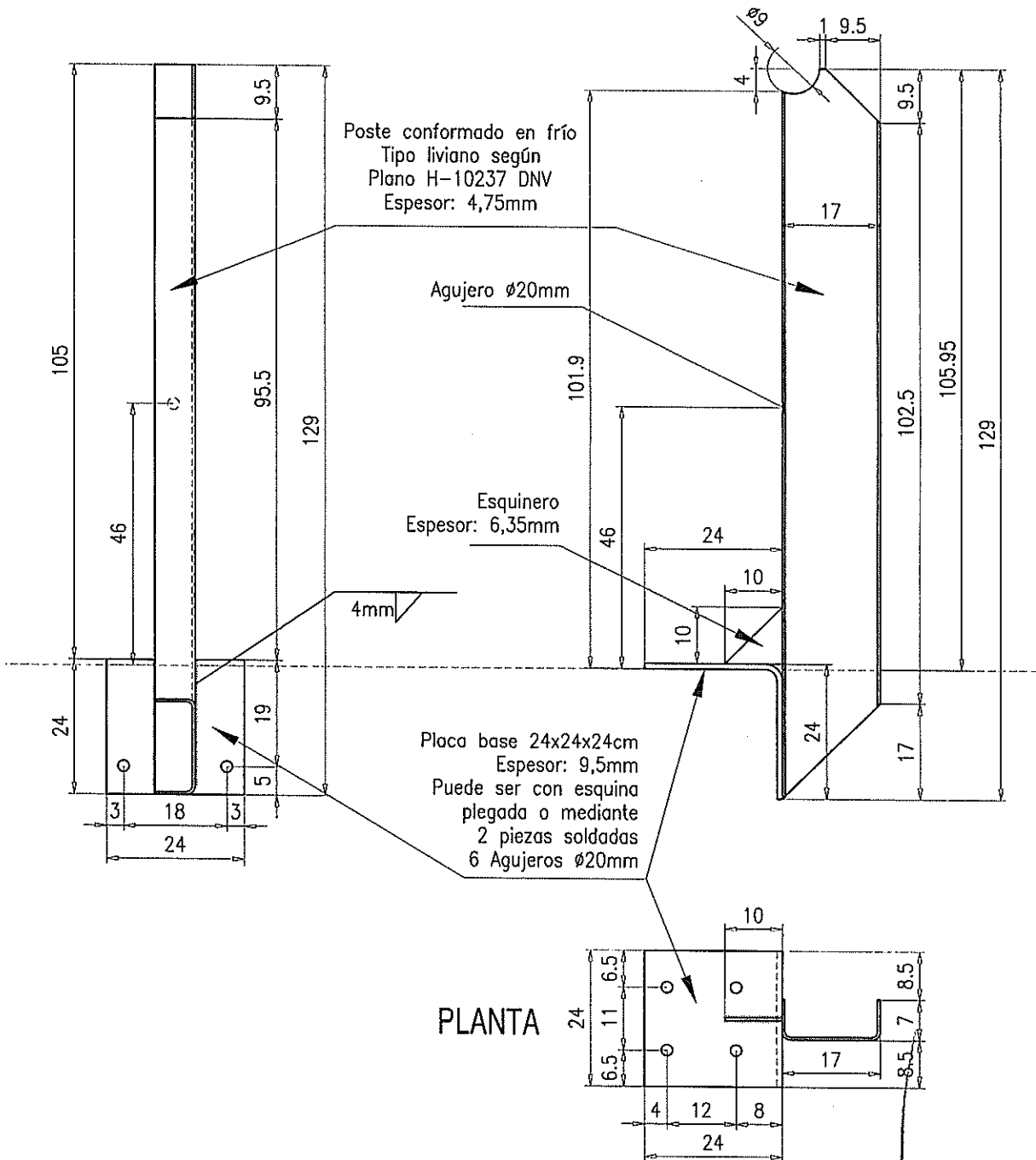
VISTA LATERAL
